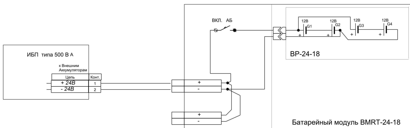
Рисунок 3 - Схема электрическая соединений
