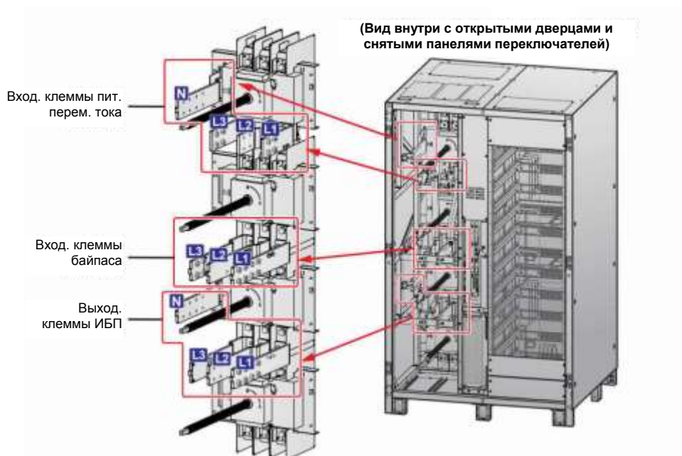
Рисунок 2-7: Клеммы: вход питания переменным током, вход байпасного питания и выход ИБП (Вид внутри с открытыми дверцами и снятыми панелями переключателей)
