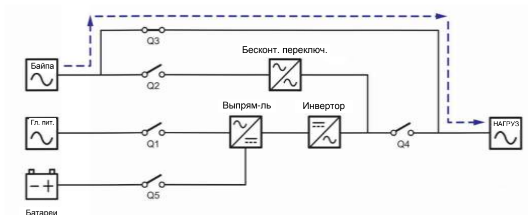
Рисунок 3-18: Схема ручного байпасного режима, подключение к двум линиям одного ИБП
