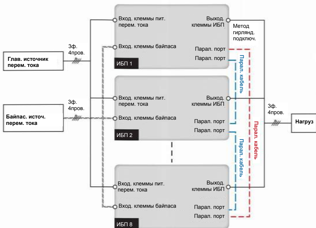
Рисунок 5-16: Схема подключения параллельных устройств к двум линиям питания
