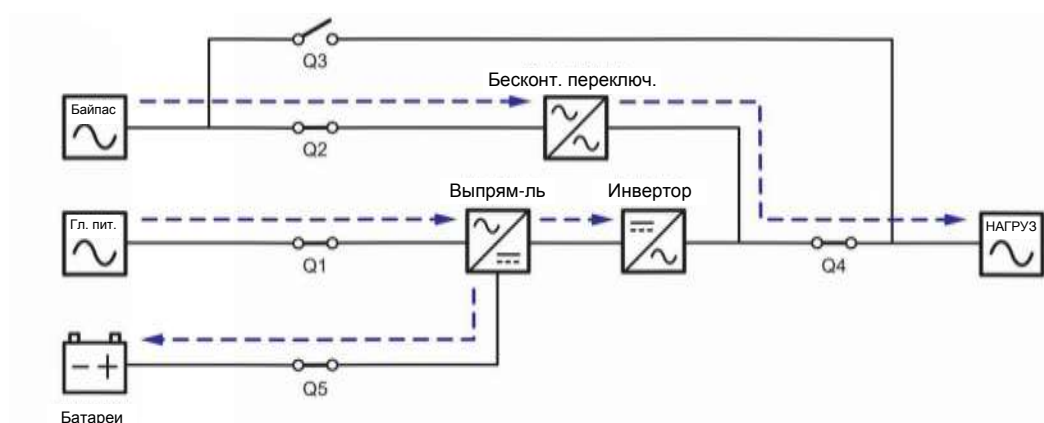
Рисунок 3-19: Схема ЕСО-режима, подключение одного ИБП к двум линиям питания
