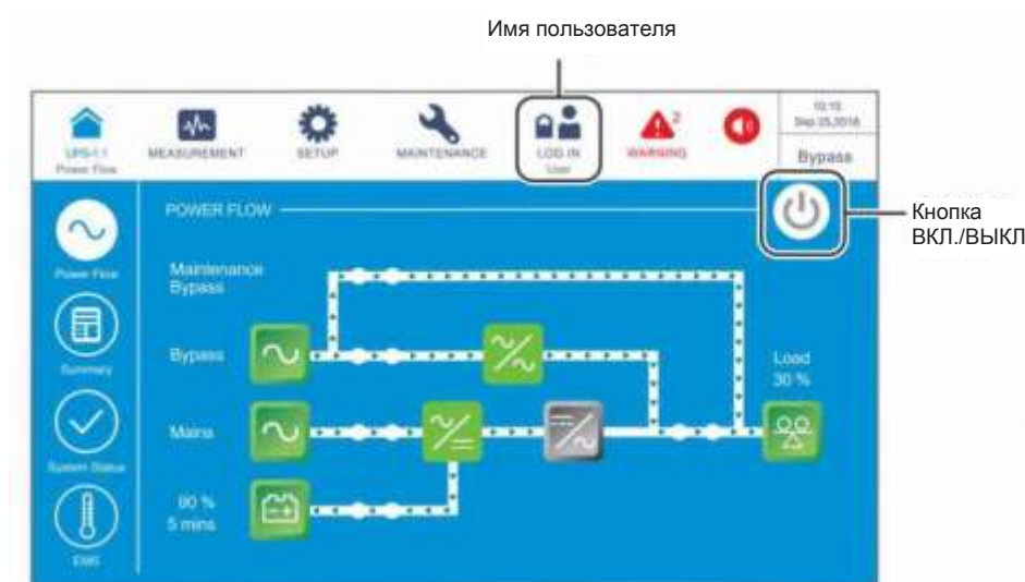
Рисунок 6-18: Экран режима байпаса: расположение кнопок имени пользователя и ВКЛ./ВЫКЛ.
