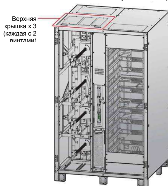
Рисунок 5-11: Расположение верхних крышек
