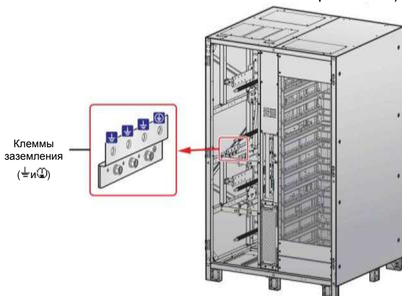
Рисунок 5-10: Клеммы заземления
