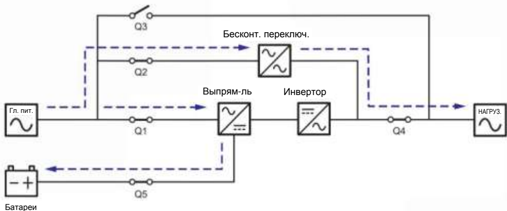
Рисунок 3-3: Схема байпасного режима, подключение одного ИБП к одной линии
