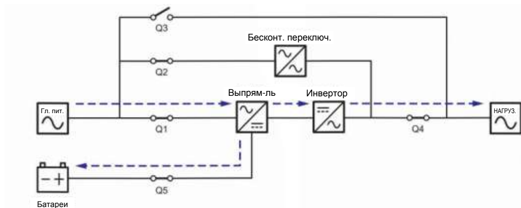
Рисунок 3-7: Схема энергосберегающего режима, подключение к одной линии одного ИБП
