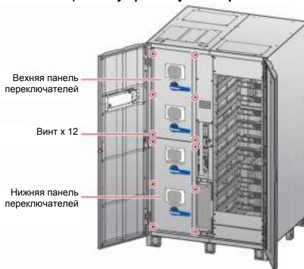
Рисунок 2-6: Расположение винтов панелей переключателей
