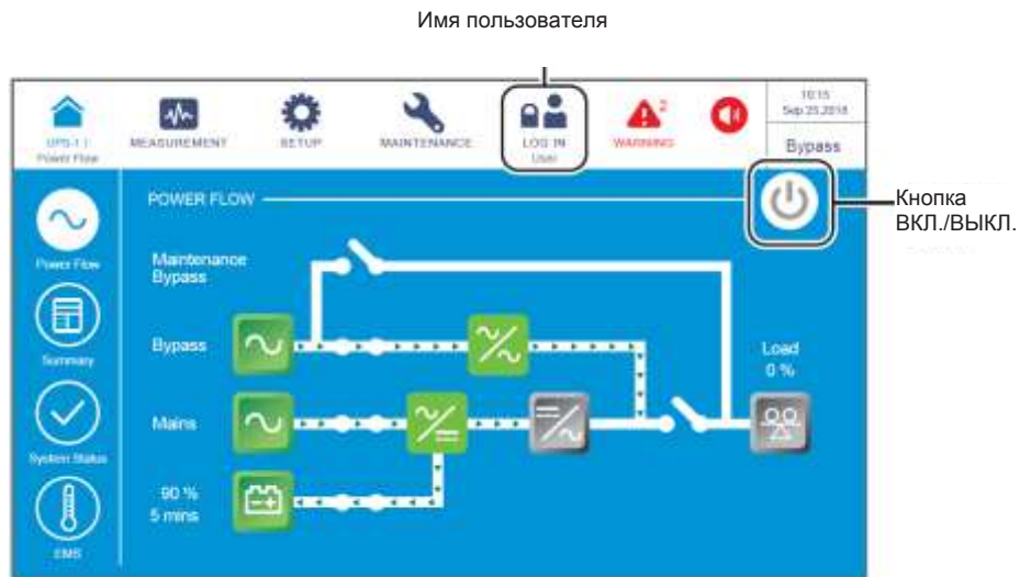
Рисунок 6-11: Главный экран: расположение кнопок имени пользователя и ВКЛ./ВЫКЛ.
