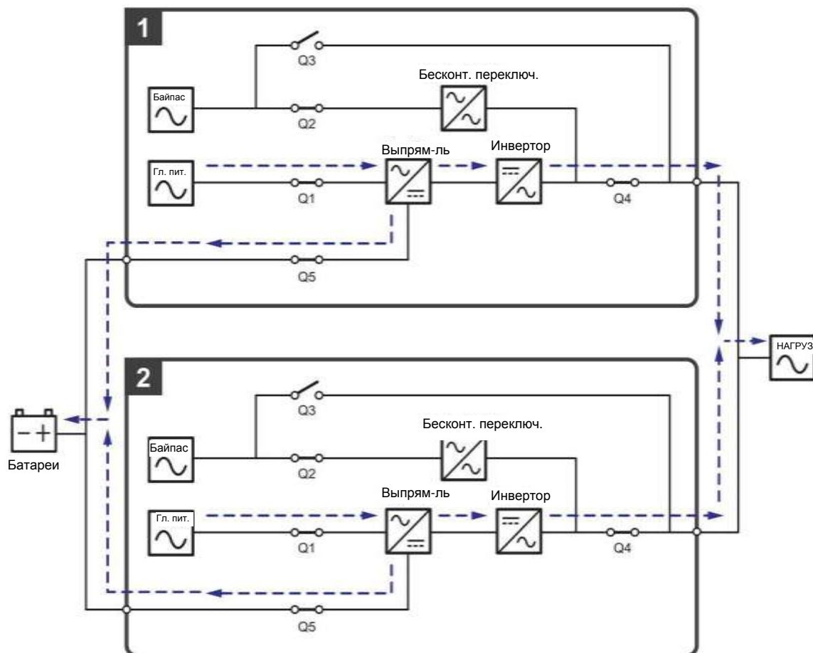
Рисунок 3-29: Схема общей батареи, только для параллельных ИБП, подсоединенных к одному внешнему батарейному модулю (модулям)
