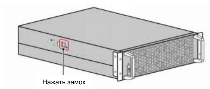
Рисунок 5-41: Нажатие на замок силового модуля
