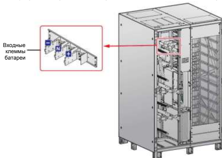
Рисунок 2-8: Клеммы: вход для подключения батарей (Вид внутри с открытыми дверцами и снятыми панелями переключателей)
