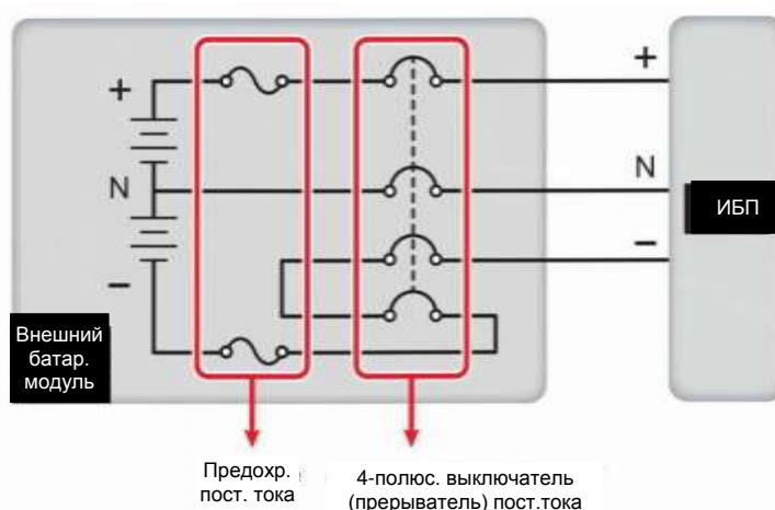
Рисунок 5-18: Установка 4-х полюсного автоматического выключателя или прерывателя постоянного тока с предохранителем
