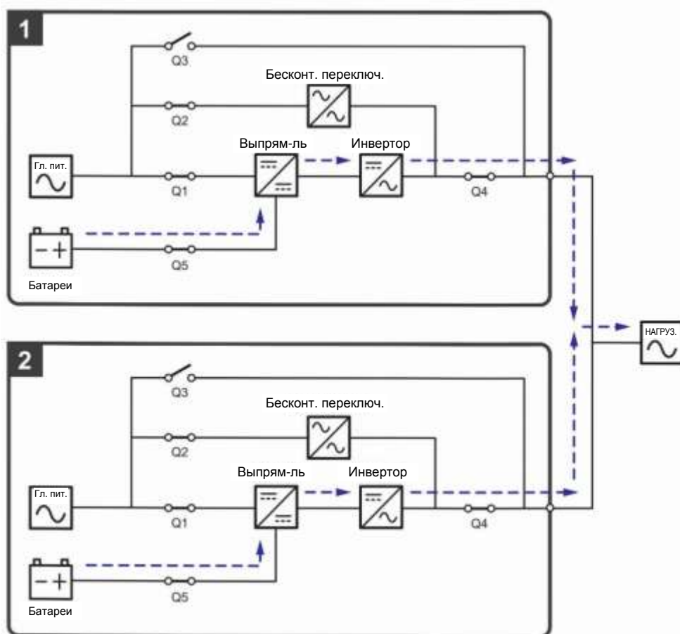
Рисунок 3-10: Схема батарейного режима, подключение параллельных ИБП к одной линии
