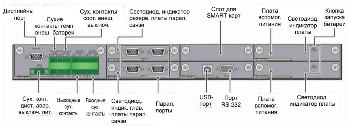
Рисунок 4-3: Функции интерфейсов связи
