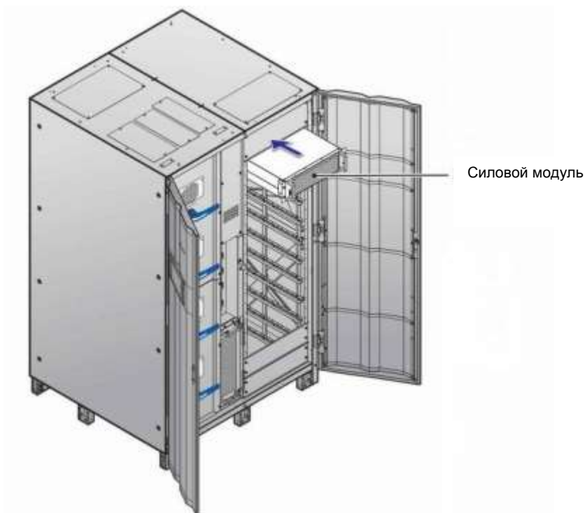
Рисунок 5-35: Установка силового модуля в ИБП
