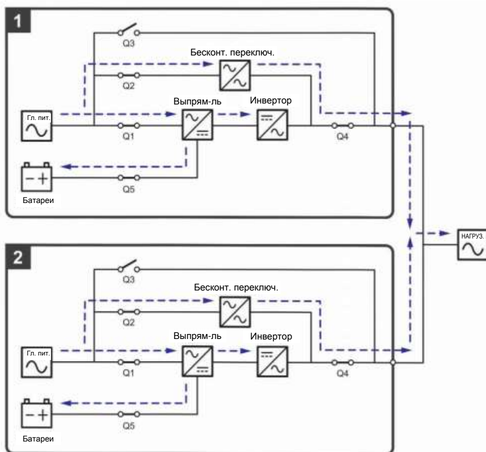
Рисунок 3-13: Схема ЕСО-режима, подключение к одной линии параллельных ИБП
