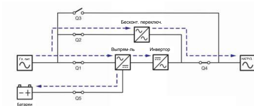
Рисунок 3-5: Схема ЕСО-режима, подключение одного ИБП к одной линии
