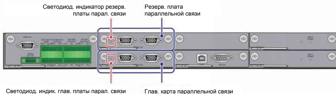
Рисунок 4-11: Расположение главной и резервной плат параллельной передачи данных и их светодиодных индикаторов
