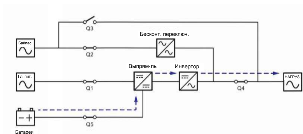
Рисунок 3-16: Схема батарейного режима, подключение одного ИБП к двум линиям питания
