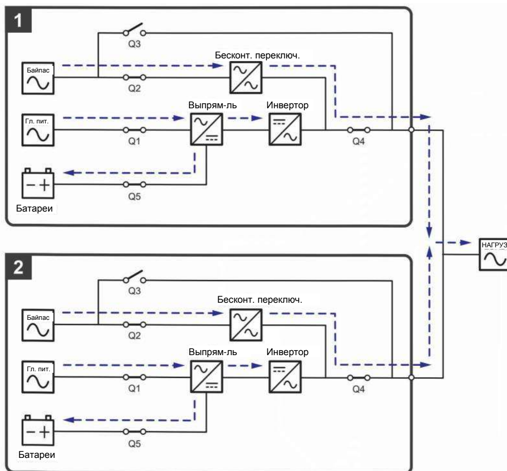
Рисунок 3-26: Схема ECO-режима, подключение к двум линиям параллельных ИБП
