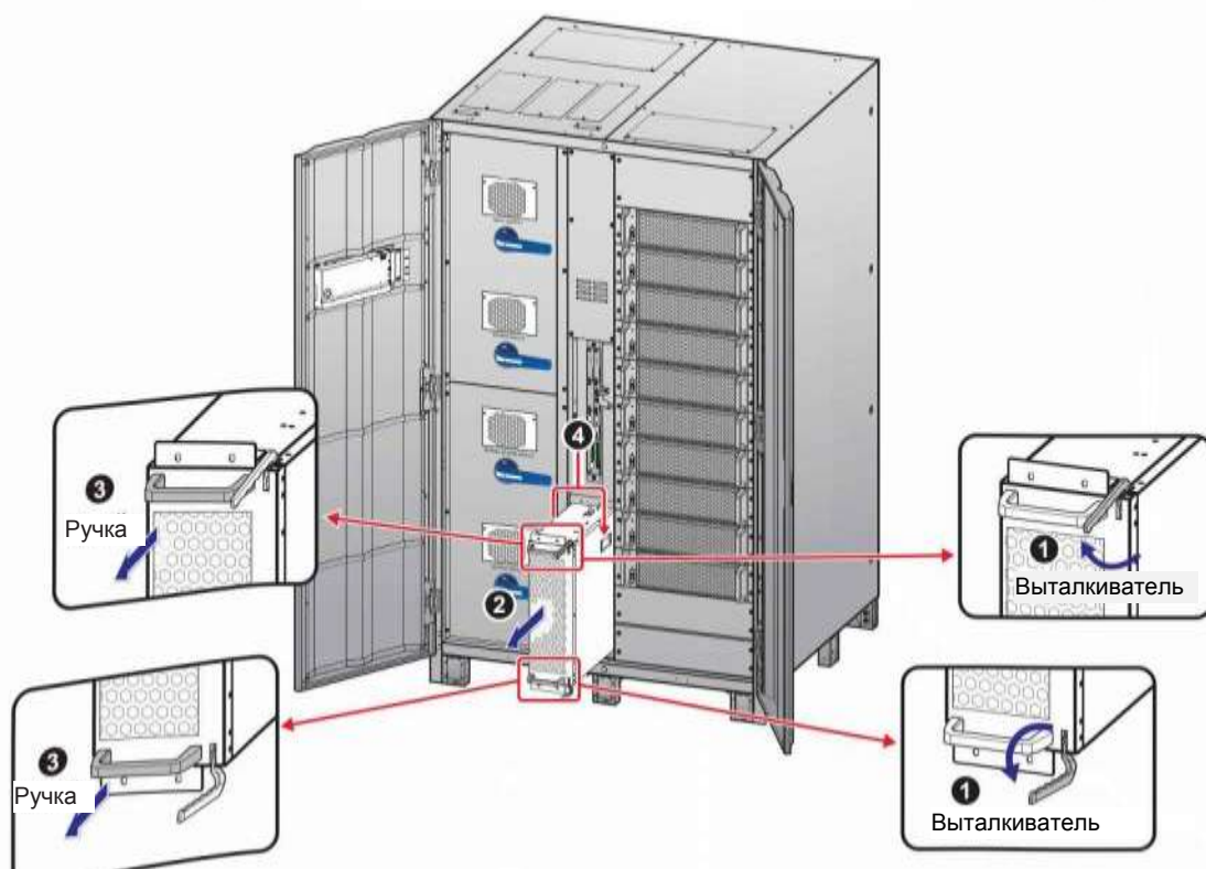
Рисунок 5-29: Демонтаж STS-модуля из шкафа ИБП
