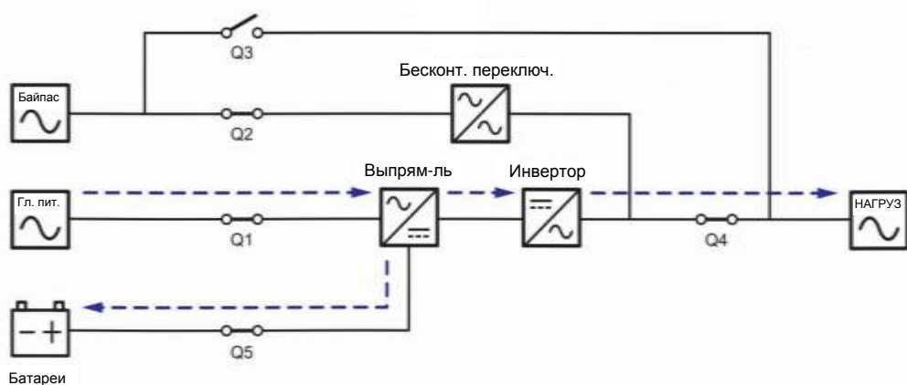
Рисунок 3-20: Схема режима преобразования частоты, подключение к двум линиям одного ИБП
