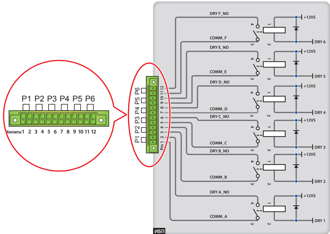
Рис. 5-4. Выходные сухие контакты: назначение и подключение выводов
