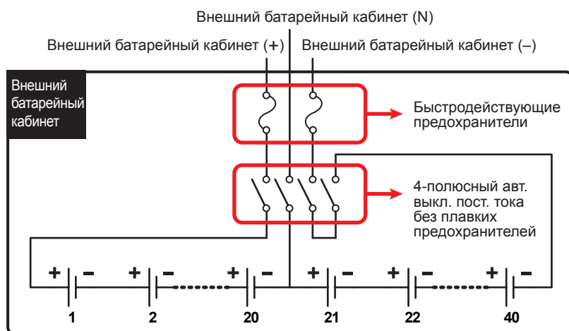
Рис. 6-20. Подключение внешнего батарейного кабинета сторонних производителей
