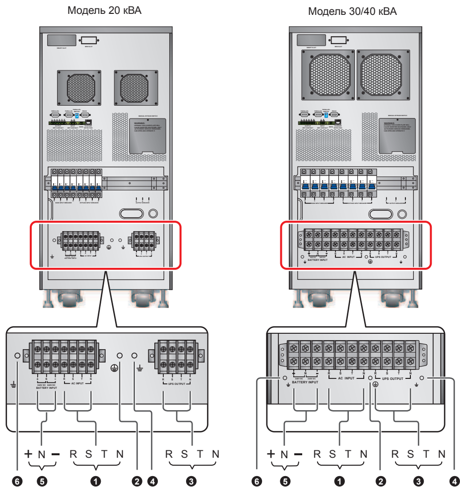
Рис. 6-8. Блок зажимов
