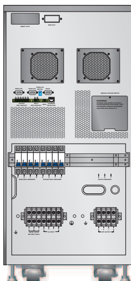
Модель 20 кВА: вид сзади
