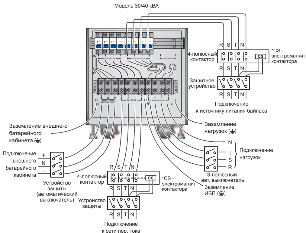
Рис. 6-13. Схема подключения I одиночного ИБП 30/40 кВА в конфигурации с двумя входами
