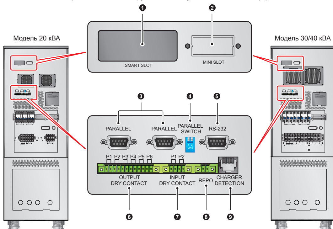
Рис. 5-1. Коммуникационные интерфейсы
